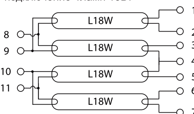
подключение 4 ламп 18Вт
